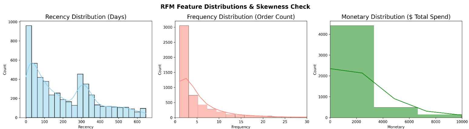
Fig: rfm_distribution
