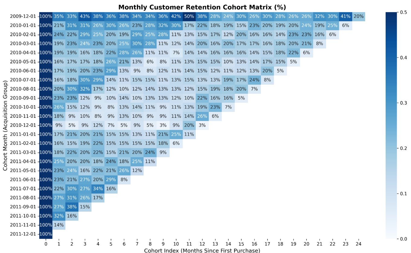
Fig: cohort_retention_heatmap
