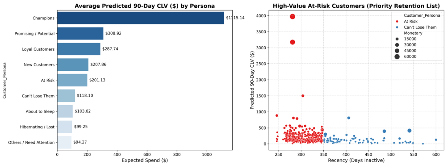
Fig: clv_evaluation_plots
